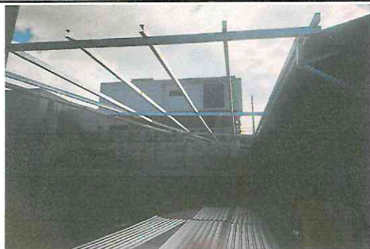
Foto 5: Sustitución de galera provisional de nylon, por galera de estructura metálica de 2.80 metros de alto, lamina troquelada calibre 26.
